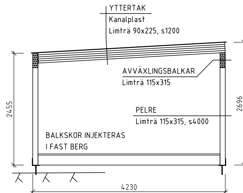
SEKTION (Teknisk beskrivning)
