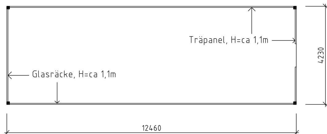
PLAN (BEFINTLIGT) 1:100
