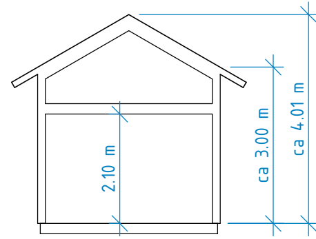
Sektion A
